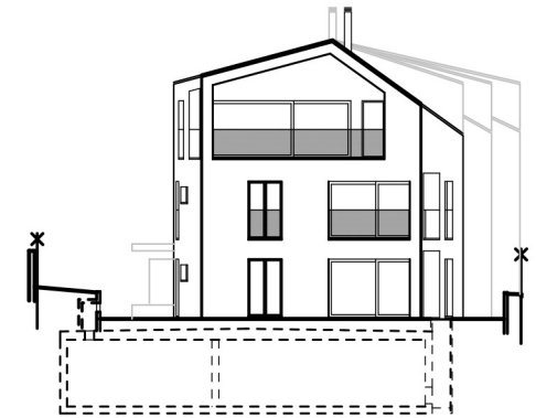
West-Fassade
