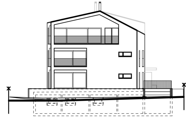
Ost-Fassade
